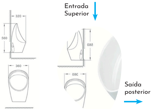
Urínol COM FLUXÓMETRO S160/224 Ref.: RSKZ223
