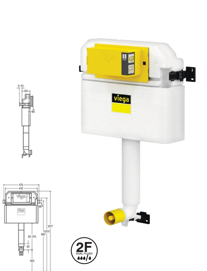
Sanita / toilette / cuvette / inodoro / wc S284/398
